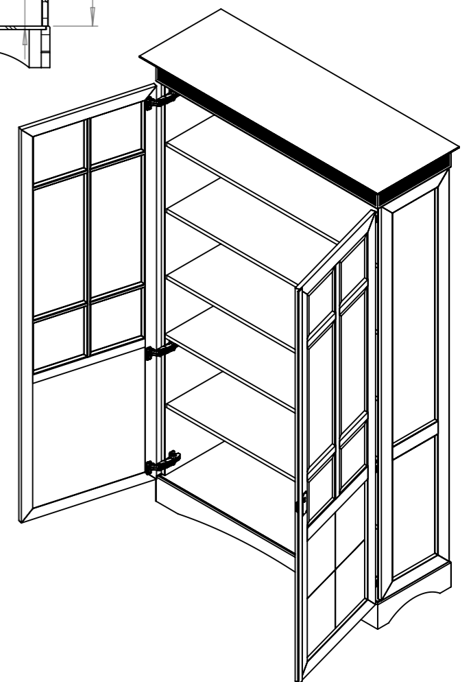
SZ1 Szafa 1300x450x2100
